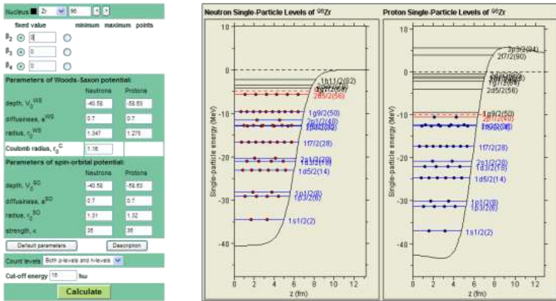
Рис. 3. Пример построения на экране монитора схемы расположения уровней с графиками потенциалов для ядра ^{96}\text{Zr} .
